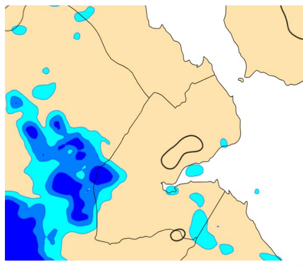
Accumulation de pluie sur 3 heures
