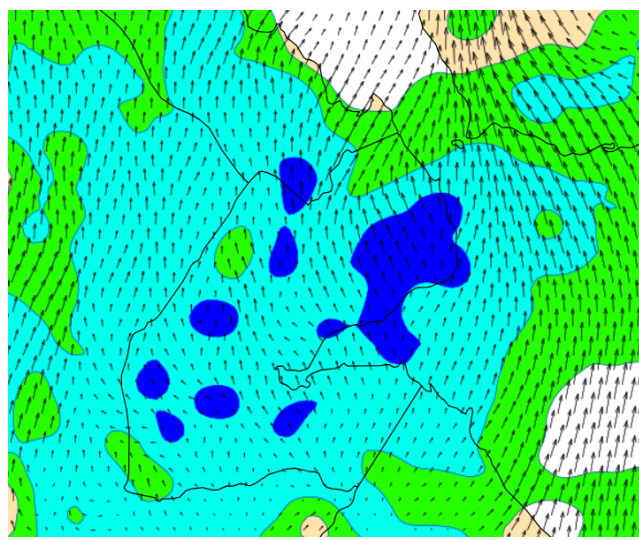
Humidité relative au niveau de 850 hPa
