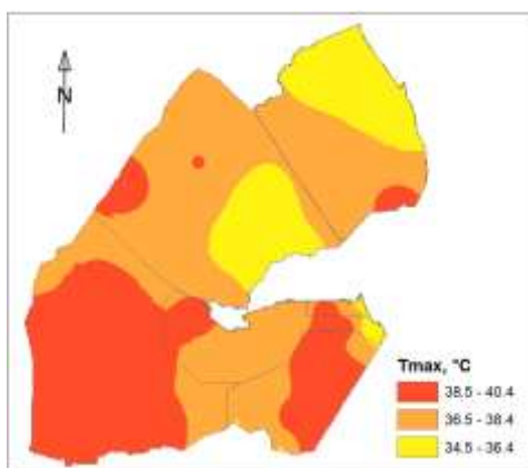
Figure 2 : Prévion de Températures maximales 01 – 08 Octobre 2025.
