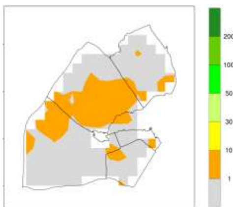
Figure 1 : Prévision des précipitations 01 – 08 Octobre 2025.
