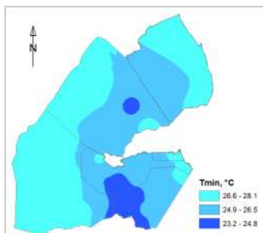
Figure 3 : Prévion de températures minimales 01 – 08 Octobre 2025.
