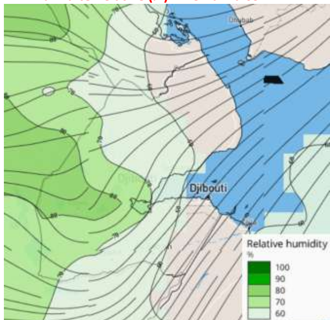
Humidité Relative (%) – Demain à 09h-12h
