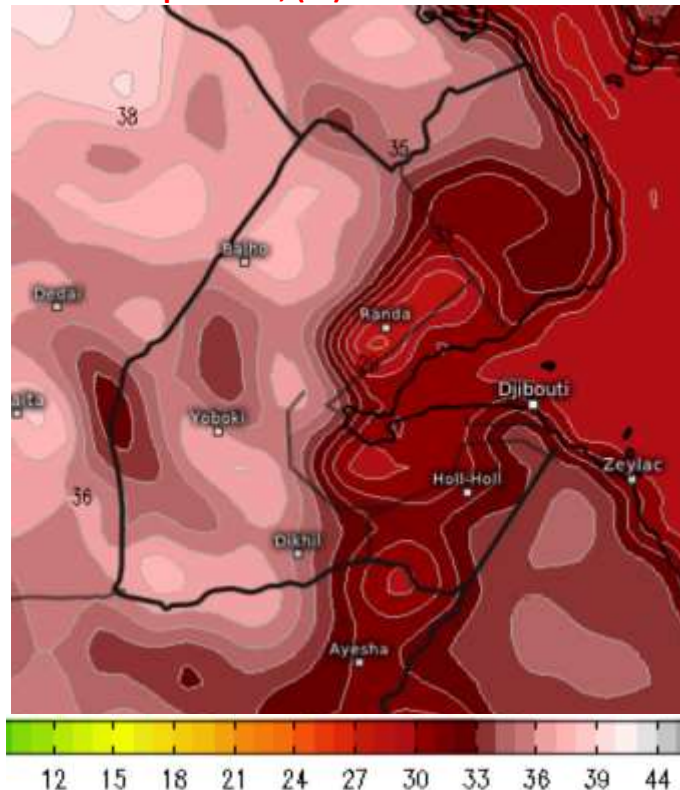
Température, (°C) – Demain à 14h00
