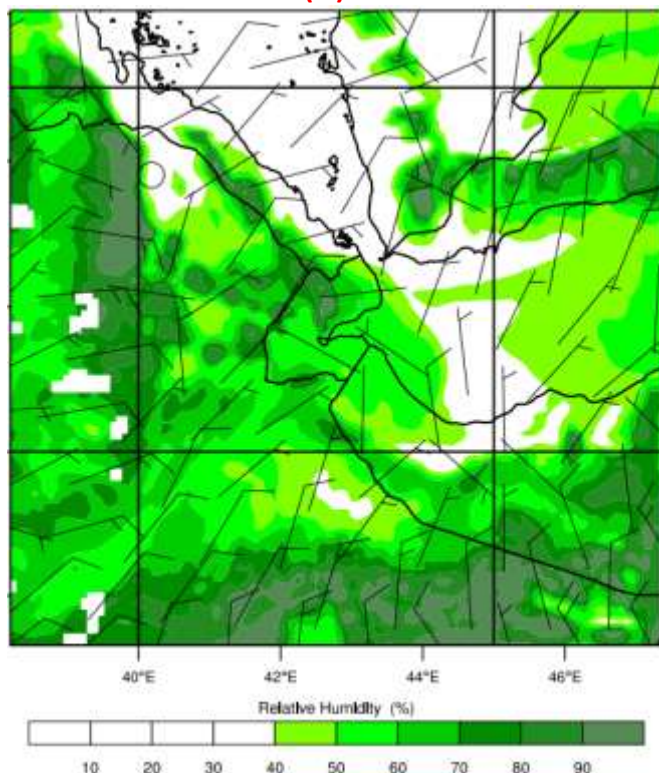
Humidité Relative (%) – Demain à 12h-15h
