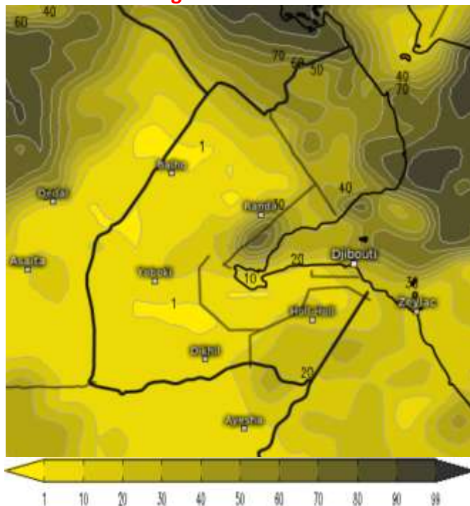
Couverture nuageuse totale – Demain à 07h00
