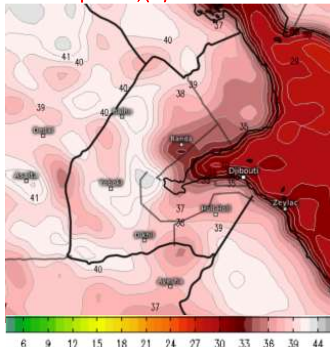
Température, (°C) – Demain à 12h00
