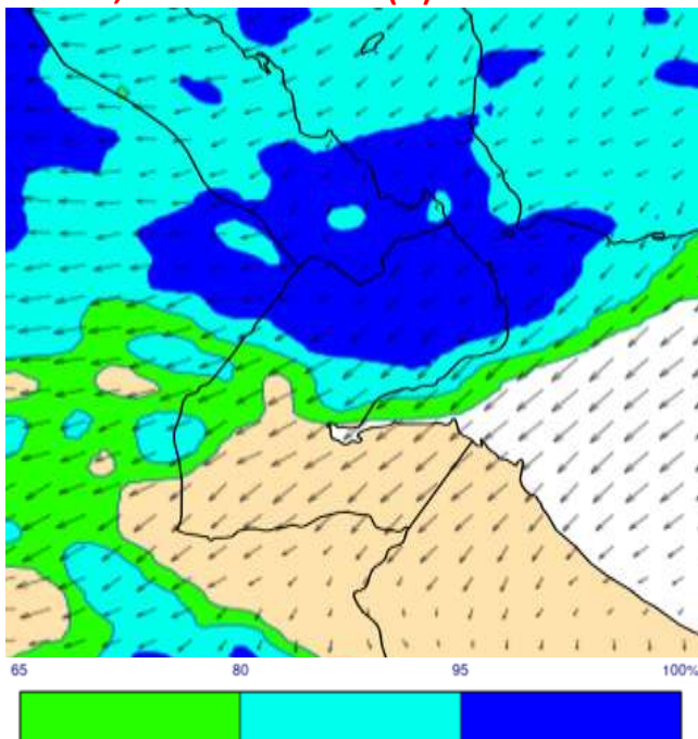
500hPa, Humidité Relative (%) – Demain à 21h00
